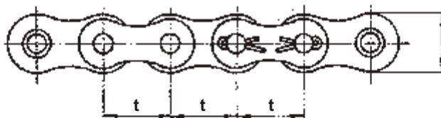
No.32 DUPLI KRIVI ČLANAK CRANKED LINK DOUBLE
